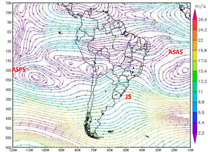
(c) Linha Corrente – 850 hPa – 21 a 31 de dezembro de 2024
