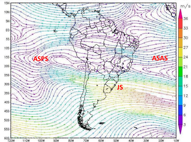
(c) Linha Corrente – 850 hPa – 01 a 10 de dezembro de 2024
