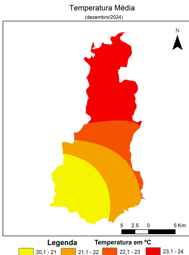
Figura 4 - Espacialização da Temperatura Média em dezembro de 2024. FONTE dos Dados: INMET e INPE
