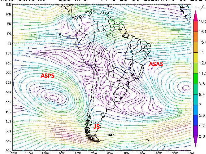
Figura 7 - Campos de Linha de Corrente 200 hPa. - (a), 500 hPa. - (b) e 850 hPa – (c), do 2º Decêndio de dezembro de 2024; demonstrando interação entre os sistemas atmosféricos: Jato Subtropical (JS), Alta da Bolívia (AB), Vórtice Ciclônico de Altos Níveis (VCAN), Anticiclone Subtropical do Atlântico Sul (ASAS) e o Anticiclone Subtropical do Pacífico Sul (ASPS).
