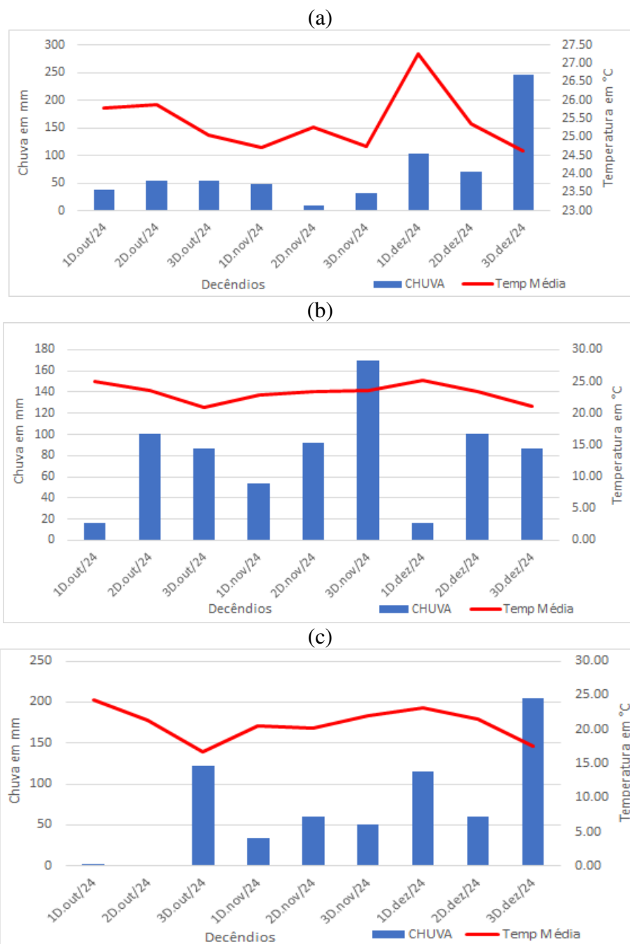
Figura 3: Histograma de Chuva e Temperatura: Caratinga (a); Timóteo (b) e PERD (c) – (outubro de 2024 e dezembro de 2024).
