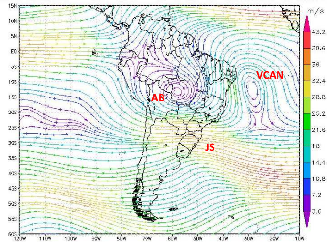
(b) Linha Corrente – 500 hPa – 21 a 31 de dezembro de 2024
