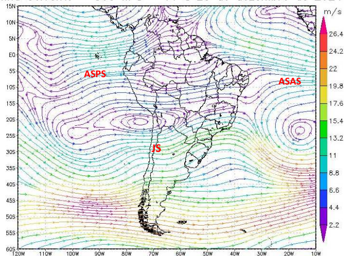
(c) Linha Corrente – 850 hPa – 11 a 20 de dezembro de 2024
