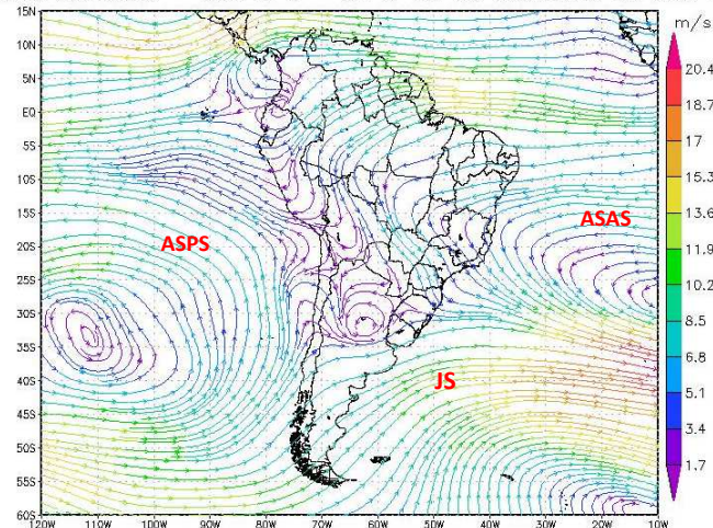
Figura 6 - Campos de Linha de Corrente 200 hPa - (a), 500 hPa - (b) e 850 hPa - (c), do 1º Decêndio de dezembro de 2024; demonstrando interação entre os sistemas atmosféricos: Jato Subtropical (JS), Alta da Bolívia (AB), Vórtice Ciclônico de Altos Níveis (VCAN), Anticiclone Subtropical do Atlântico Sul (ASAS) e o Anticiclone Subtropical do Pacífico Sul (ASPS).
