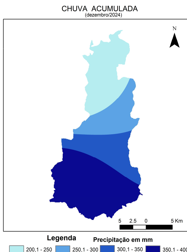
Figura 5 - Espacialização da Chuva da Acumulada em dezembro de 2024. FONTE dos Dados: INMET e INPE
