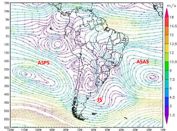
Figura 8 - Campos de Linha de Corrente 200 hPa- (a), 500 hPa - (b) e 850 hPa – (c), do 3º Decêndio de dezembro de 2024; demonstrando interação entre os sistemas atmosféricos: Jato Subtropical (JS), Alta da Bolívia (AB), Vórtice Ciclônico de Altos Níveis (VCAN), Anticiclone Subtropical do Atlântico Sul (ASAS) e Anticiclone Subtropical do Pacífico Sul (ASPS).
