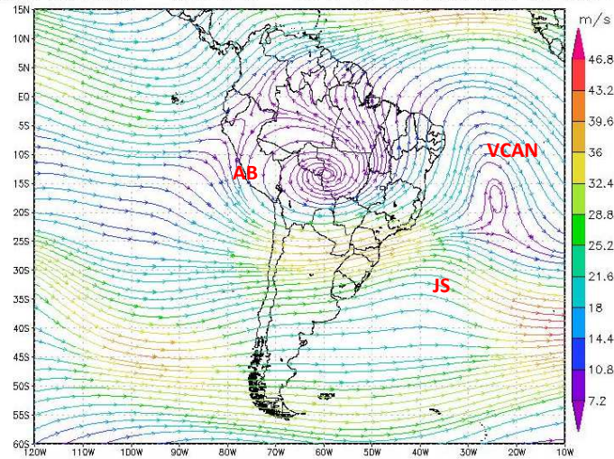
(b) Linha Corrente – 500 hPa – 11 a 20 de dezembro de 2024
