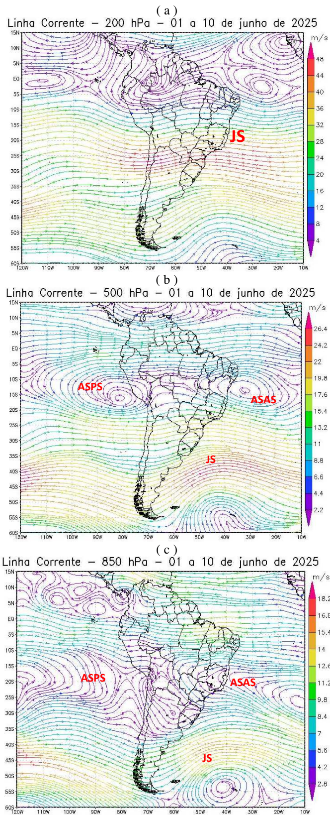
Figura 6 - Campos de Linha de Corrente 200 hPa. - (a), 500 hPa. - (b) e 850 hPa - (c), do 1º Decêndio de junho de 2025; demonstrando interação entre os sistemas atmosféricos: Jato Subtropical (JS), Anticiclone Subtropical do Atlântico Sul (ASAS) e o Anticiclone Subtropical do Pacífico Sul (ASPS). FONTE - Dados: NOAA 2025.
