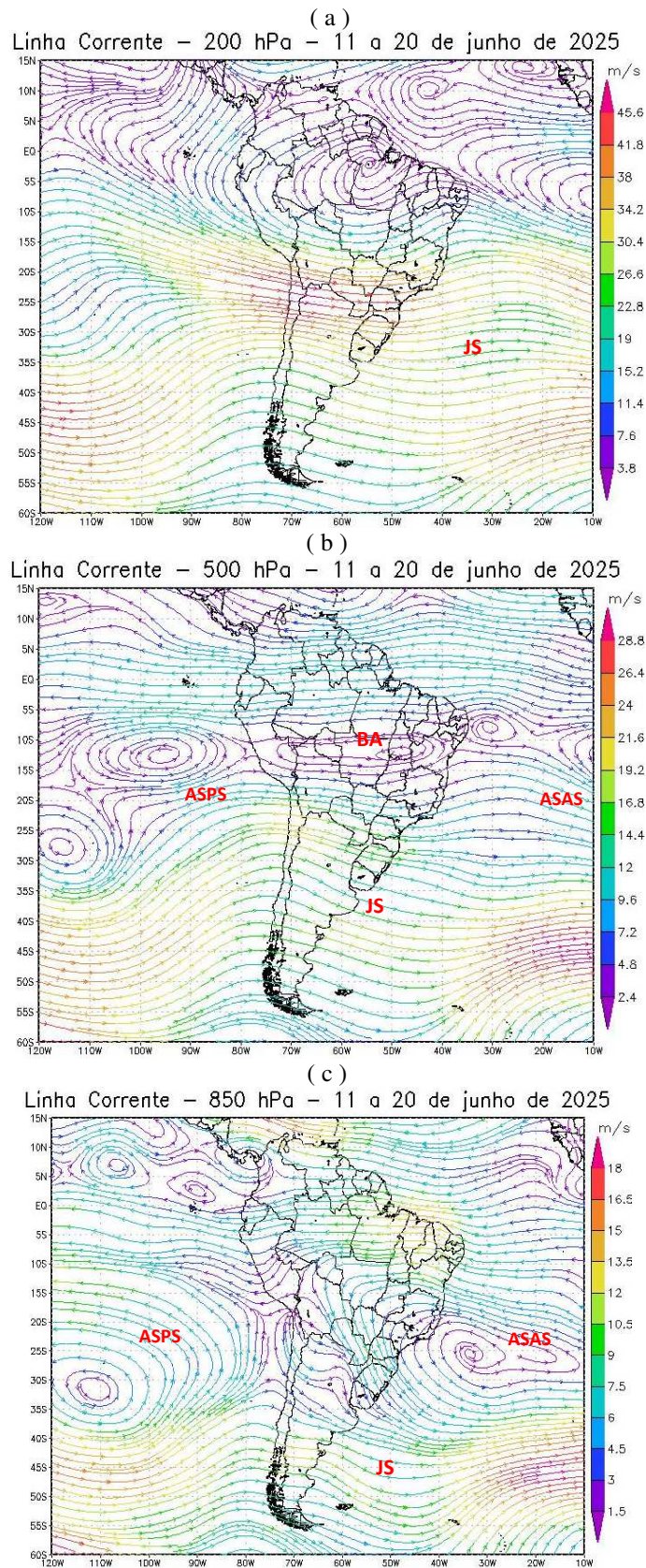
Figura 7 - Campos de Linha de Corrente 200 hPa. - (a), 500 hPa - (b) e 850 hPa - (c), do 2º Decêndio de junho de 2025; demonstrando interação entre os sistemas atmosféricos: Jato Subtropical (JS), Bloqueio Atmosférico (BA), Anticiclone Subtropical do Atlântico Sul (ASAS) e o Anticiclone Subtropical do Pacífico Sul (ASPS). FONTE - Dados: NOAA 2025.
