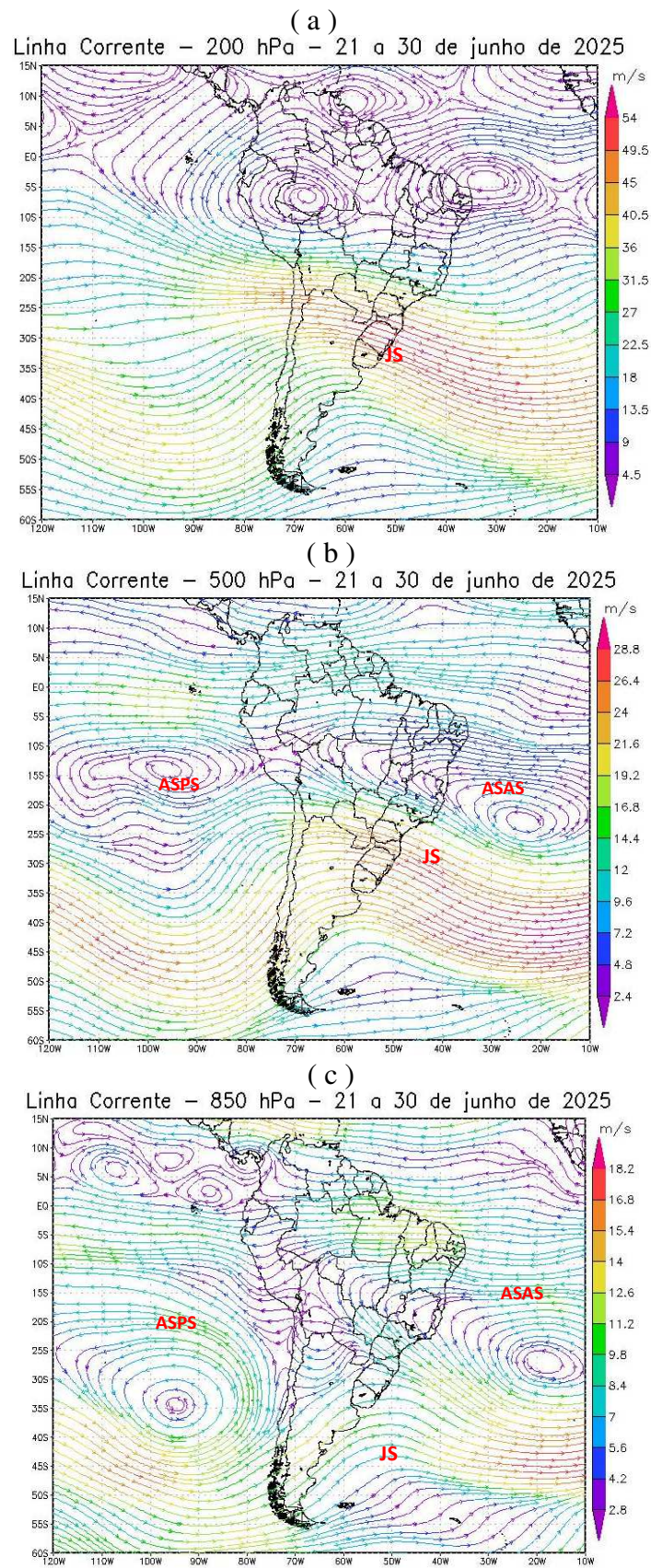
Figura 8 - Campos de Linha de Corrente 200 hPa - (a), 500 hPa - (b) e 850 hPa - (c), do 3º Decêndio de junho de 2025; demonstrando interação entre os sistemas atmosféricos: Jato Subtropical (JS), Anticiclone Subtropical do Atlântico Sul (ASAS) e Anticiclone Subtropical do Pacífico Sul (ASPS).
