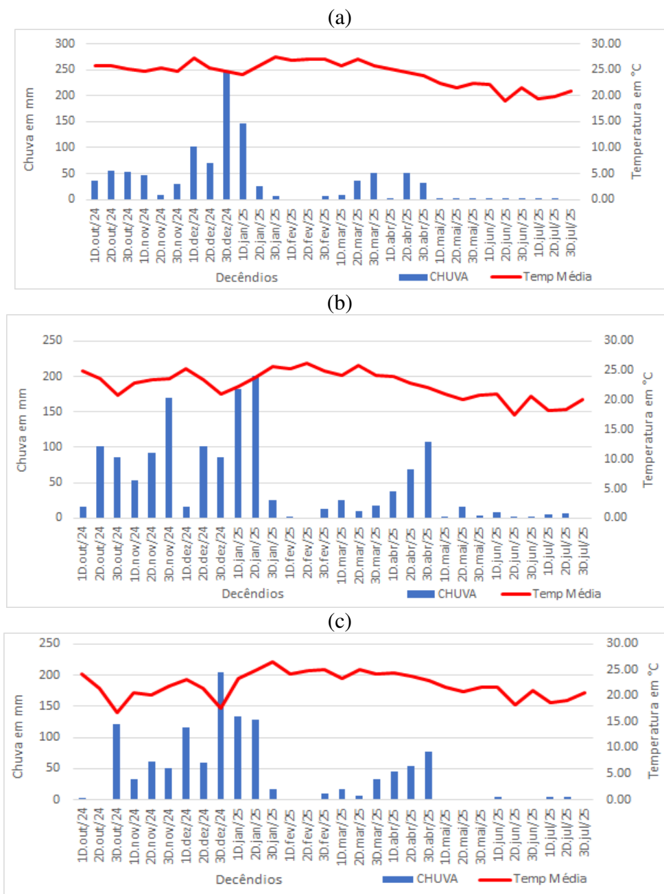
Figura 3: Histograma de Chuva e Temperatura: Caratinga (a); Timóteo (b) e PERD (c) – (outubro de 2024 a julho de 2025).
