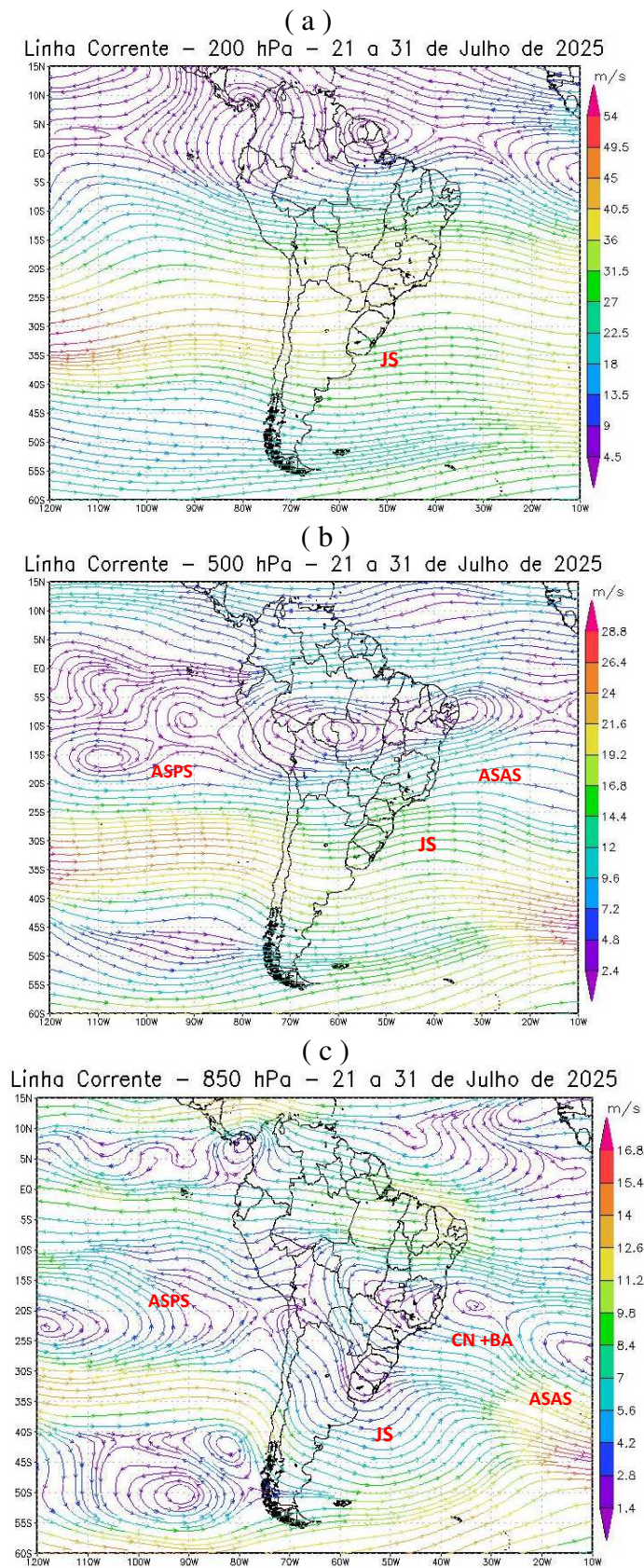
Figura 8 - Campos de Linha de Corrente 200 hPa - (a), 500 hPa - (b) e 850 hPa - (c), do 3º Decêndio de julho de 2025; demonstrando interação entre os sistemas atmosféricos: Jato Subtropical (JS), Cavado do Nordeste (CN) + Bloqueio Atmosférico (BA), Anticiclone Subtropical do Atlântico Sul (ASAS) e Anticiclone Subtropical do Pacífico Sul (ASPS). FONTE - Dados: NOAA 2025.
