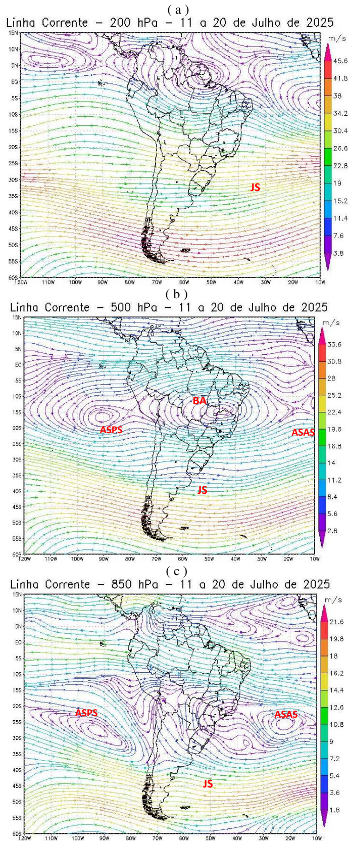
Figura 7 - Campos de Linha de Corrente 200 hPa. - (a), 500 hPa. - (b) e 850 hPa - (c), do 2º Decêndio de julho de 2025; demonstrando interação entre os sistemas atmosféricos: Jato Subtropical (JS), Bloqueio Atmosférico (BA), Anticiclone Subtropical do Atlântico Sul (ASAS) e o Anticiclone Subtropical do Pacífico Sul (ASPS). FONTE - Dados: NOAA 2025.
