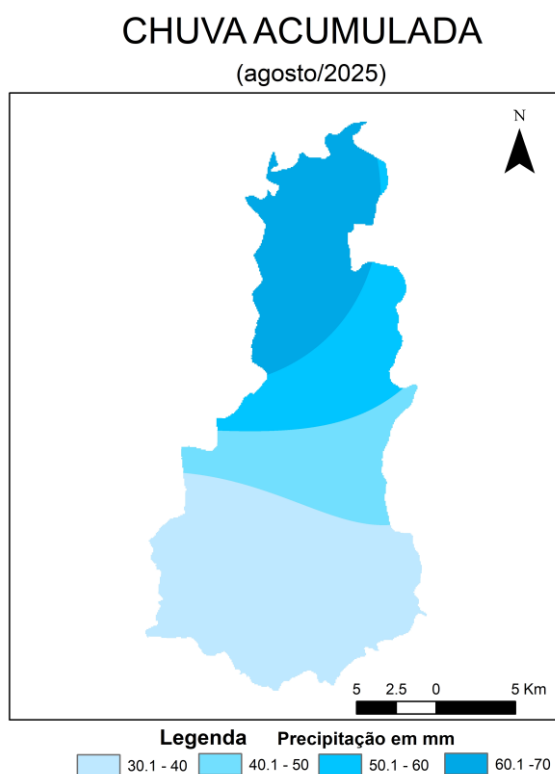
Figura 5 - Espacialização da Chuva da Acumulada em agosto de 2025. FONTE dos Dados: INMET e INPE
