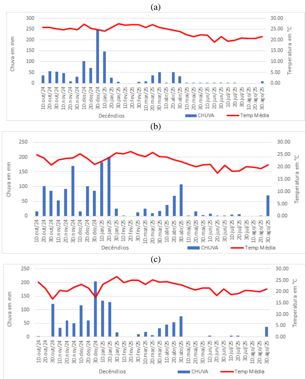
Figura 3: Histograma de Chuva e Temperatura: Caratinga (a); Timóteo (b) e PERD (c) – (outubro de 2024 a agosto de 2025).
