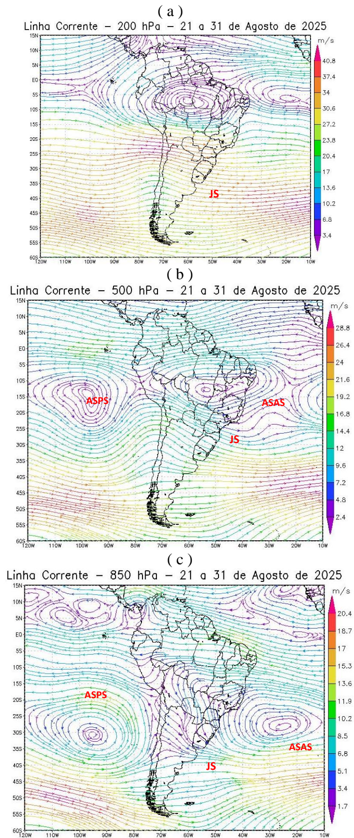
Figura 8 - Campos de Linha de Corrente 200 hPa - (a), 500 hPa - (b) e 850 hPa - (c), do 3º Decêndio de agosto de 2025; demonstrando interação entre os sistemas atmosféricos: Jato Subtropical (JS), Anticiclone Subtropical do Atlântico Sul (ASAS) e Anticiclone Subtropical do Pacífico Sul (ASPS).
