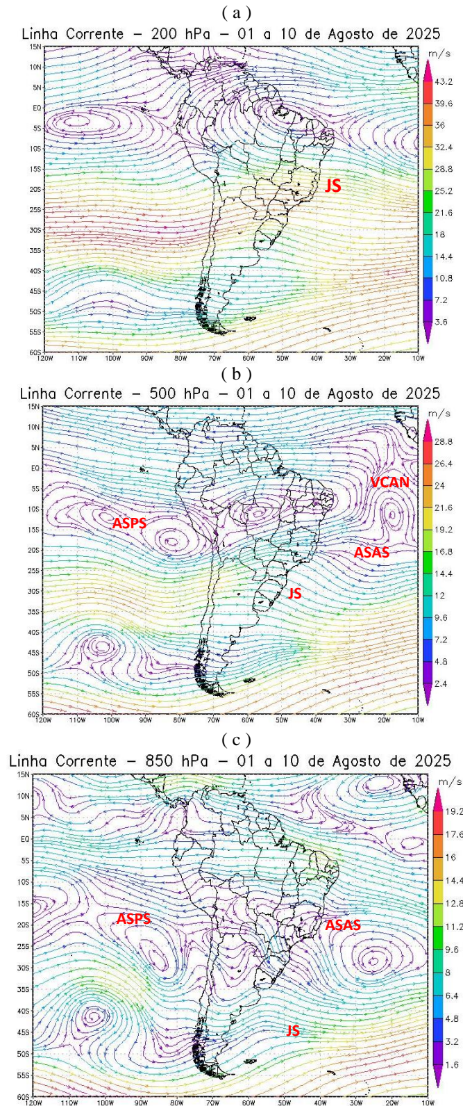
Figura 6 - Campos de Linha de Corrente 200 hPa. - (a), 500 hPa. - (b) e 850 hPa – (c), do 1º Decêndio de agosto de 2025; demonstrando interação entre os sistemas atmosféricos: Jato Subtropical (JS), Vórtice Ciclônico de Altos Níveis (VCAN), Anticiclone Subtropical do Atlântico Sul (ASAS) e o Anticiclone Subtropical do Pacífico Sul (ASPS). FONTE - Dados: NOAA 2025.
