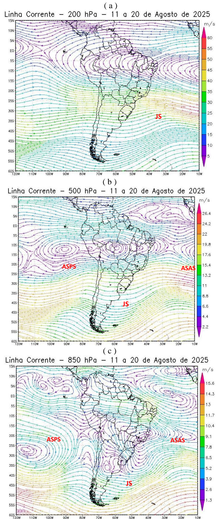
Figura 7 - Campos de Linha de Corrente 200 hPa. - (a), 500 hPa. - (b) e 850 hPa – (c), do 2º Decêndio de agosto de 2025; demonstrando interação entre os sistemas atmosféricos: Jato Subtropical (JS), Anticiclone Subtropical do Atlântico Sul (ASAS) e o Anticiclone Subtropical do Pacífico Sul (ASPS).
